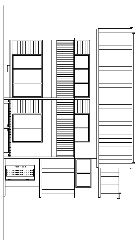
南立面図
